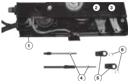
Рис. 12 Подключение тросов к блоку дистанционного управления
